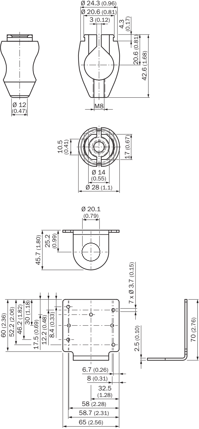
尺寸图 (尺寸单位: mm)
