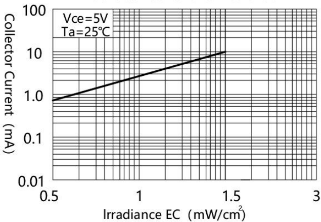
集电极电流与辐射强度的关系
