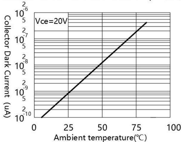
集电极暗电流与环境温度的关系
