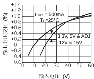
电源调整率
