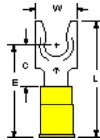
MNG10-14FL 1/4 12-10
