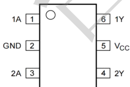
SOT363
