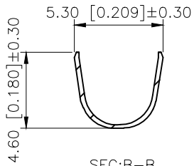
SEC:B-B
