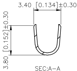
SEC:A-A
