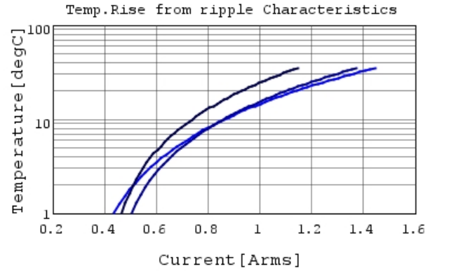
GQM1875G2E9R1CB12 Temp.rise 700MHz
