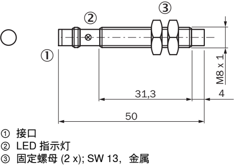
尺寸图 (尺寸单位: mm)
