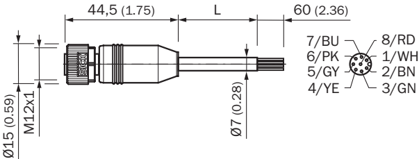
尺寸图 (尺寸单位: mm)
