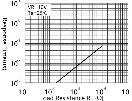
响应时间与负载电阻的关系 Response Time VS Load Resistance
