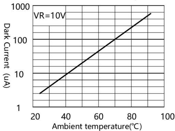
暗电流与环境温度的关系 Dark Current VS Ambient Temperature
