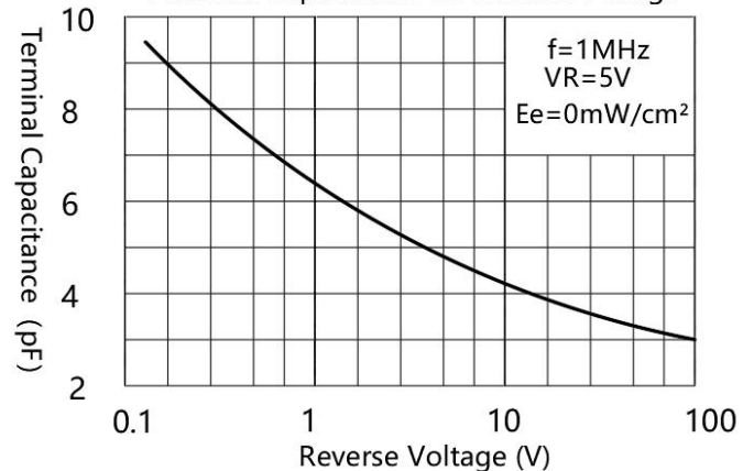
电容与反向电压的关系 Terminal Capacitance VS Reverse Voltage
