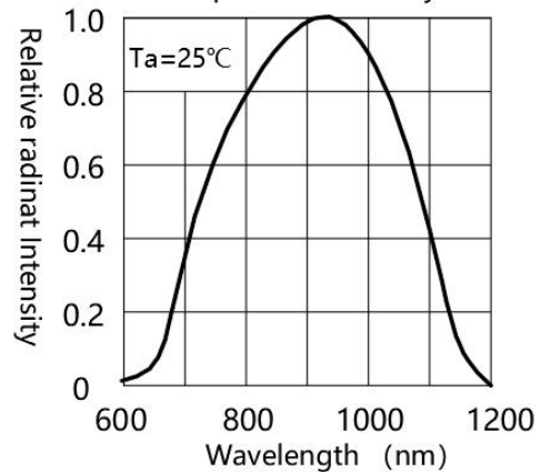
感应波长曲线图 Spectral Sensitivity
