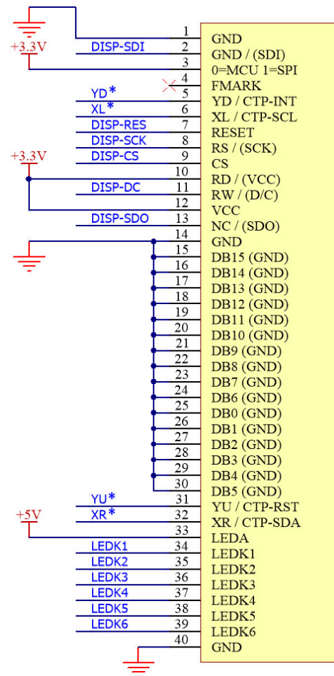
SPI Mode
