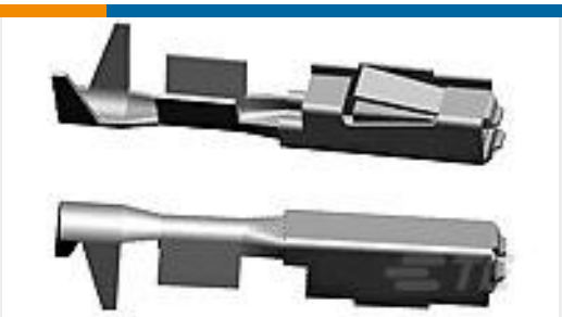
TE Part #5-928999-5 MQS0,63 Au rec LL unseal. >0,2-0,35
