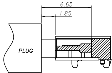
公母对插后尺寸
