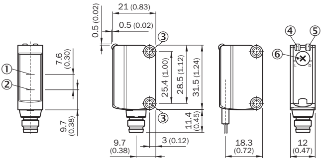
尺寸图 (尺寸单位: mm)
