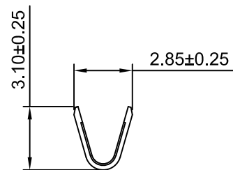
SEC:B-B
