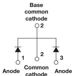
D²PAK (TO-263AB)
