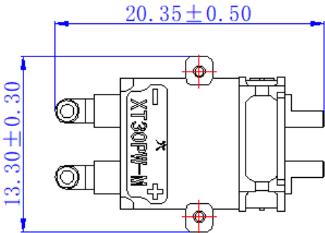
互配尺寸
