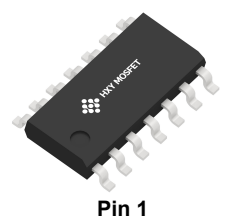
SOP-14(SOIC-14)
