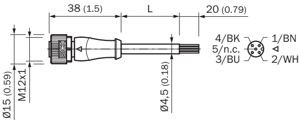
尺寸图 (尺寸单位: mm)
