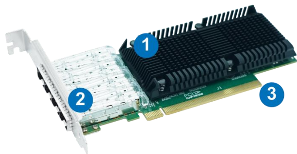
产品布局图
