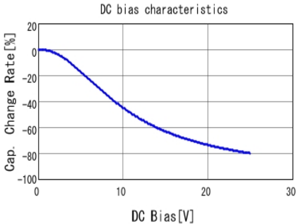
■ GRM188R61E684KA75 C-DC bias capchange, 25.0degC, AC1.
