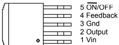
TO263-5L
