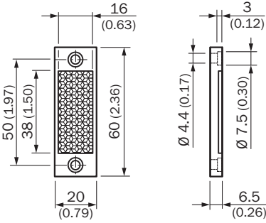
尺寸图 (尺寸单位: mm)
