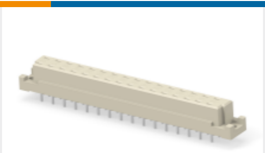
TE Part #354647-E STVD 32 F AC GG 7-02 0606 4,5 * 247 E 17
