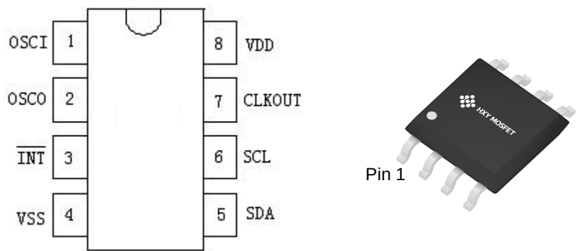
图 3. 引脚图
