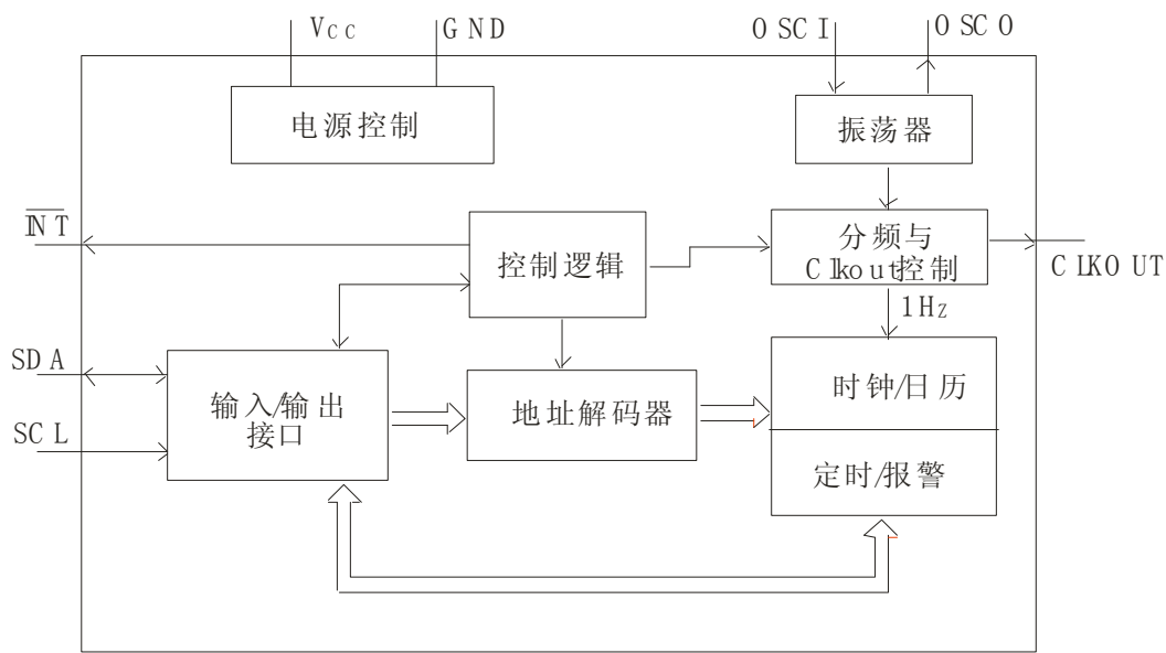
图 2. 方框图
