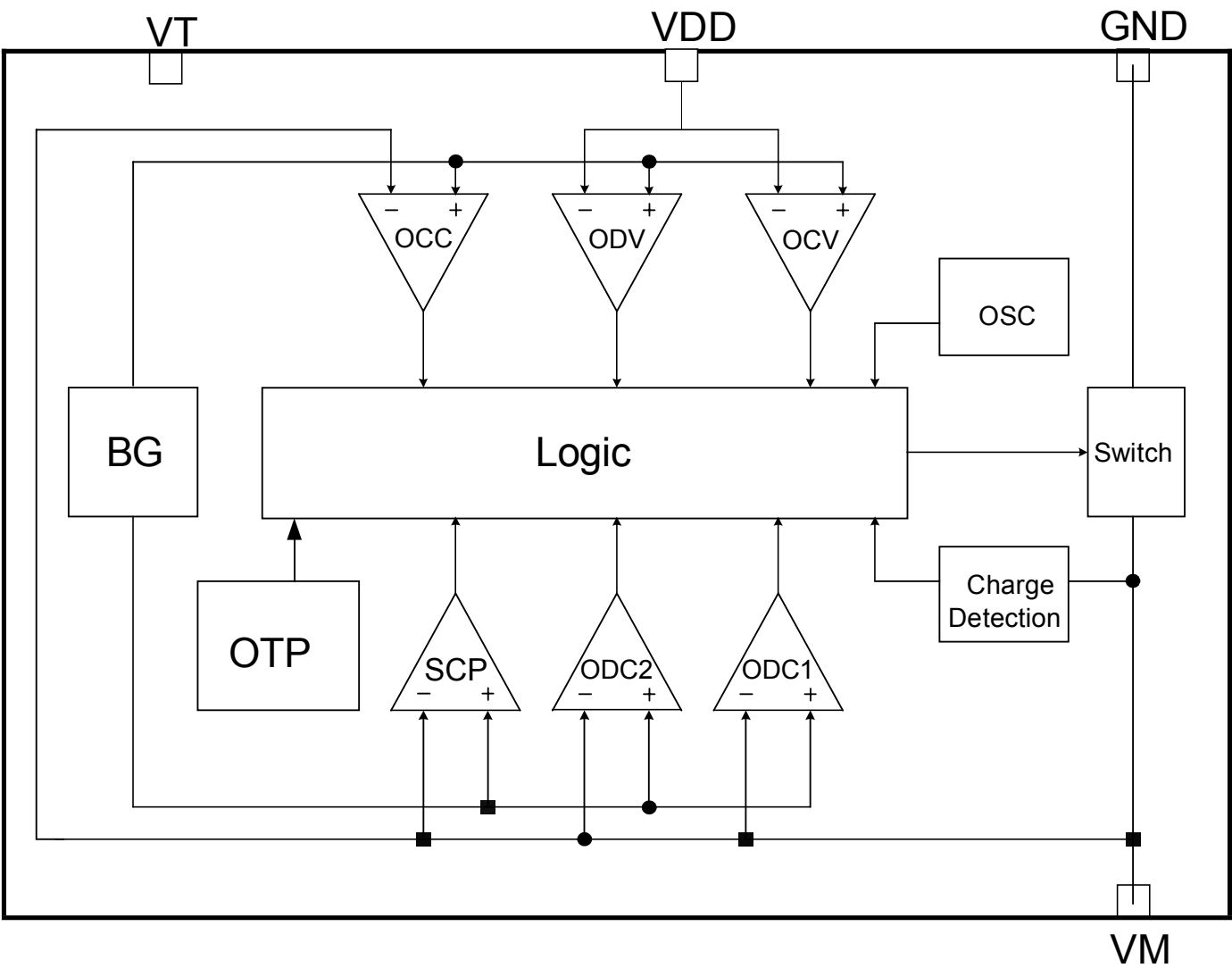
功能框图
