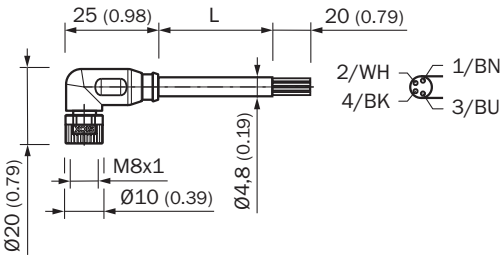
尺寸图 (尺寸单位: mm)
