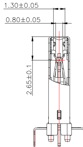
SECTION:B-B
