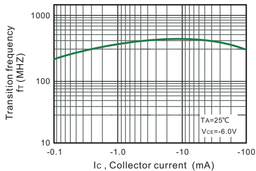
Fig.7 ft--Ic
