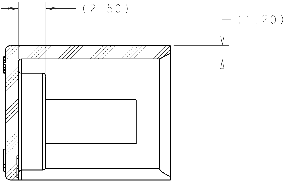
SECTION D-D
