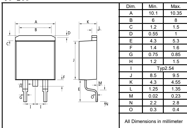
T0-263
