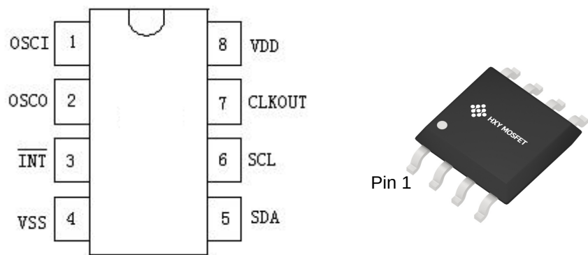
图 3. 引脚图
