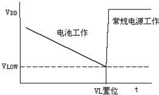
图8. 掉电检测
