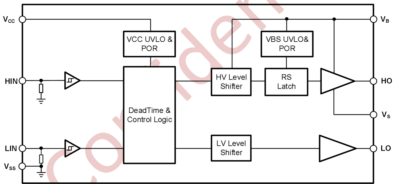
图 10-1 G2021 功能框图
