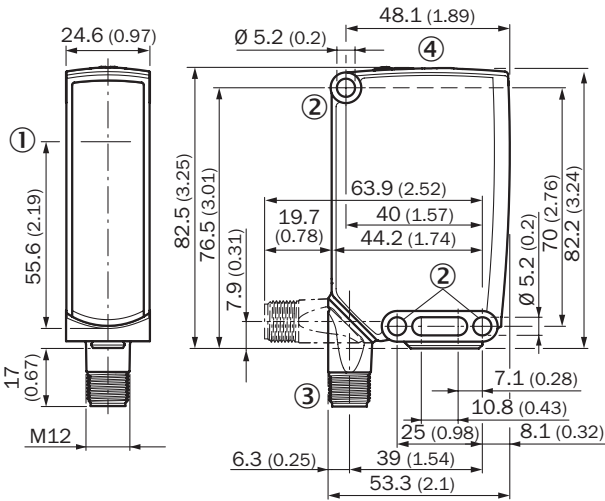
感测器尺寸圖
