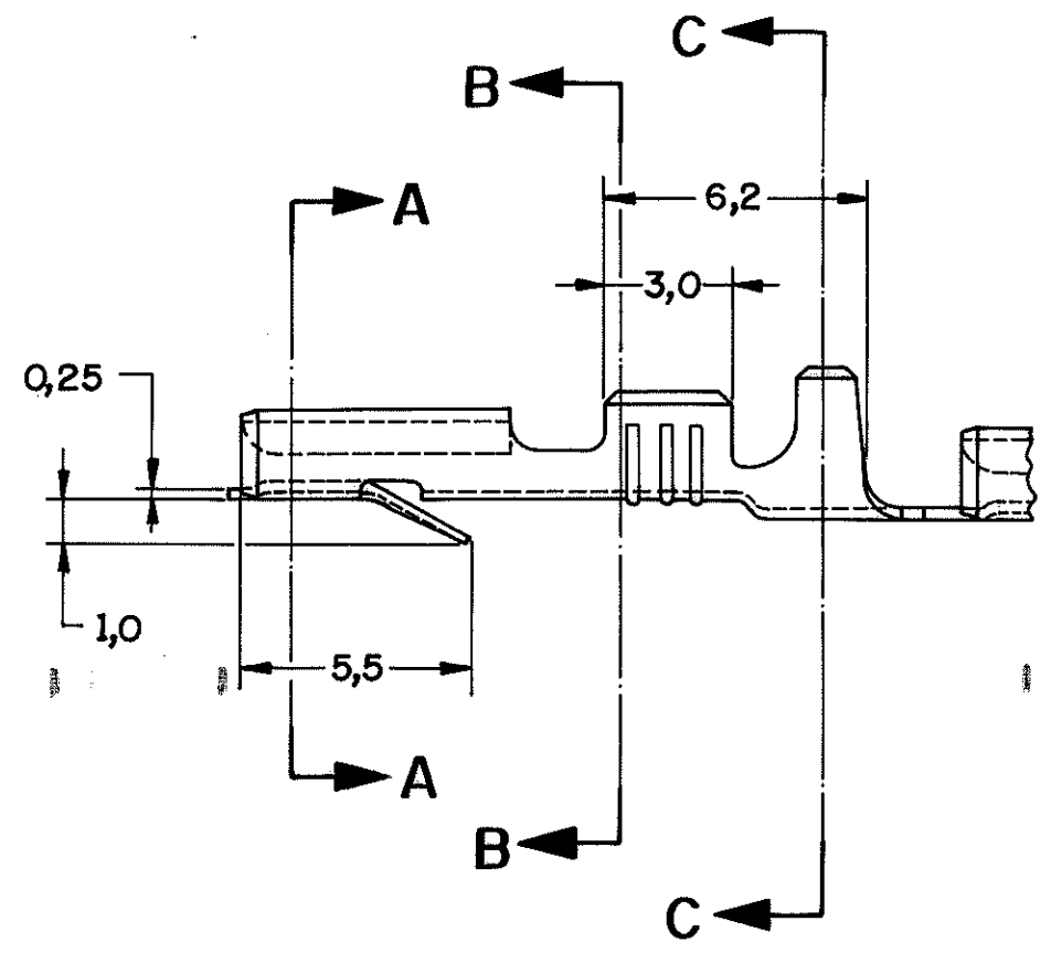
CORTE A-A SECTION
