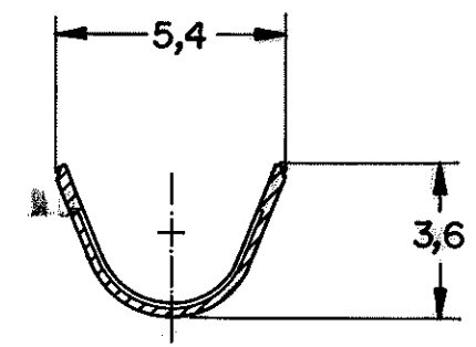
CORTE C-C SECTION
