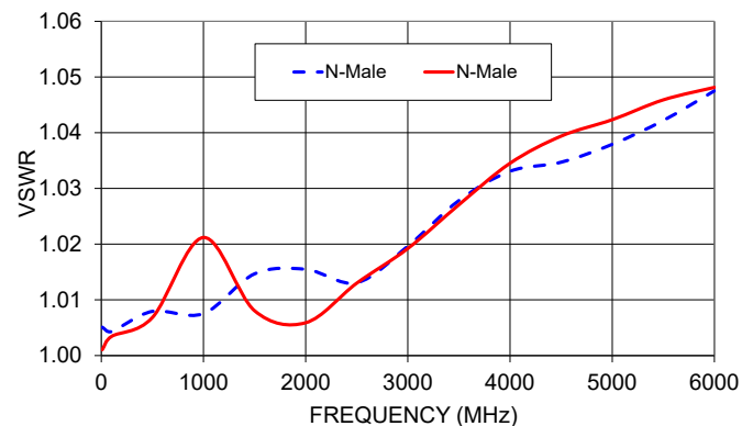
NM-NM50+ VSWR
