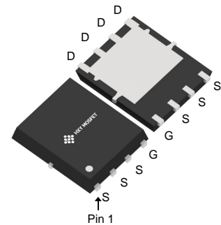
DFN5X6-8L (PowerPAK-SO-8)
