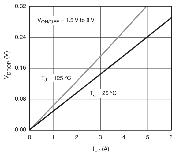
V_{DROP} vs. I_L at V_{IN} = 4.5\text{ V}
