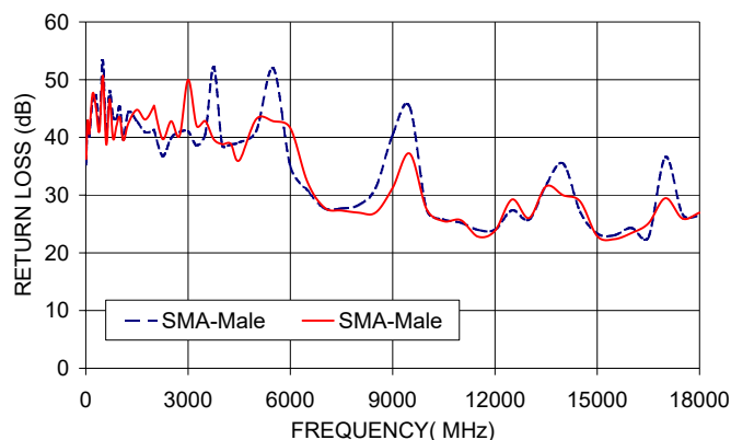
086-18SM+ RETURN LOSS
