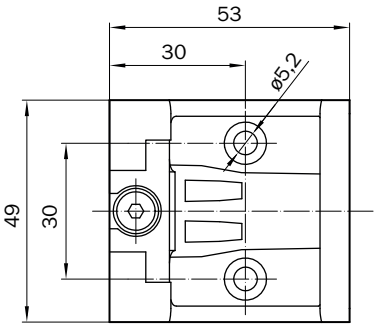
尺寸图 (尺寸单位: mm)
