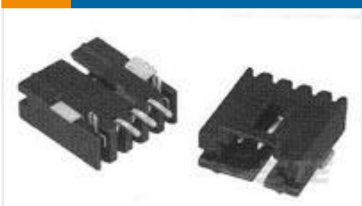
TE Part #6-147323-1 12 MTE HDR SRRA SMT.100CL
