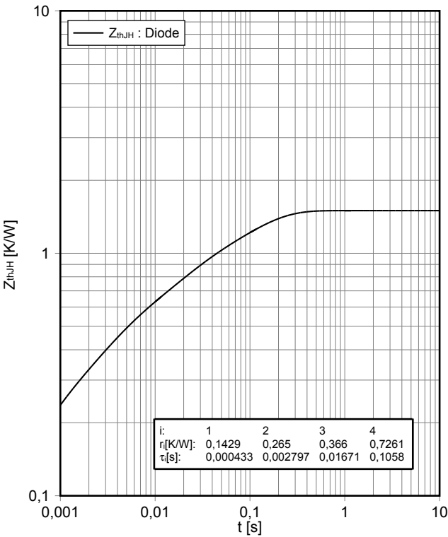
Transienter Wärmewiderstand Diode, Hochsetzsteller transient thermal impedance Diode, Boost Z_{thJH} = f(t)
