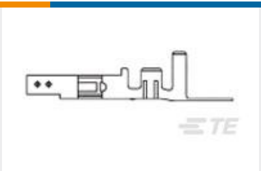
TE Part #1586055-1 VAL-U-LOK SKT BR SN 16AWG
