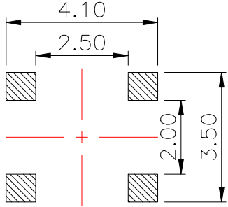
PCB.焊接图
