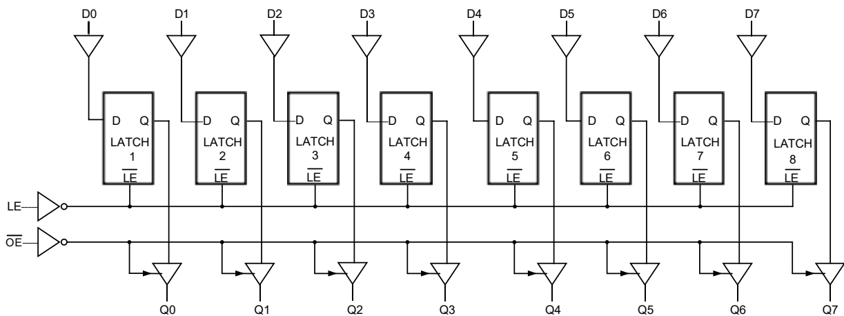
图 4 逻辑框图
