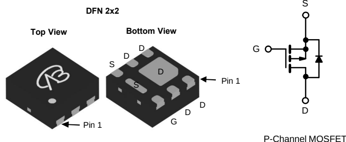
P-Channel MOSFET
