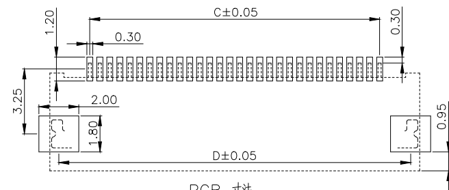
PCB 寸法 PCB Layout
