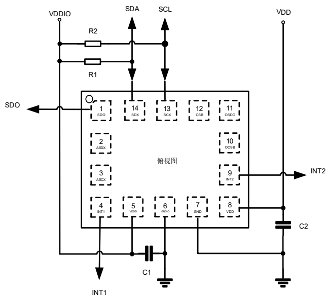
IIC通信方式连接原理图
