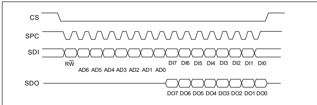
SPI读写时序
