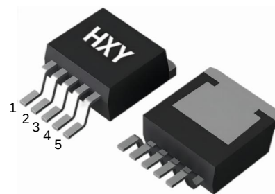
TO-263-5L (TO-263-5)
