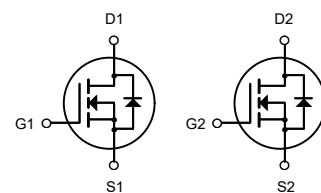
DFN3X3-8L (PDFNWB-8(3x3))
